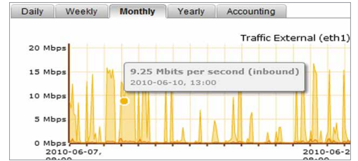
Netzwerkauslastungs-Report
