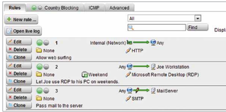
Übersicht über Paketfilterregeln
